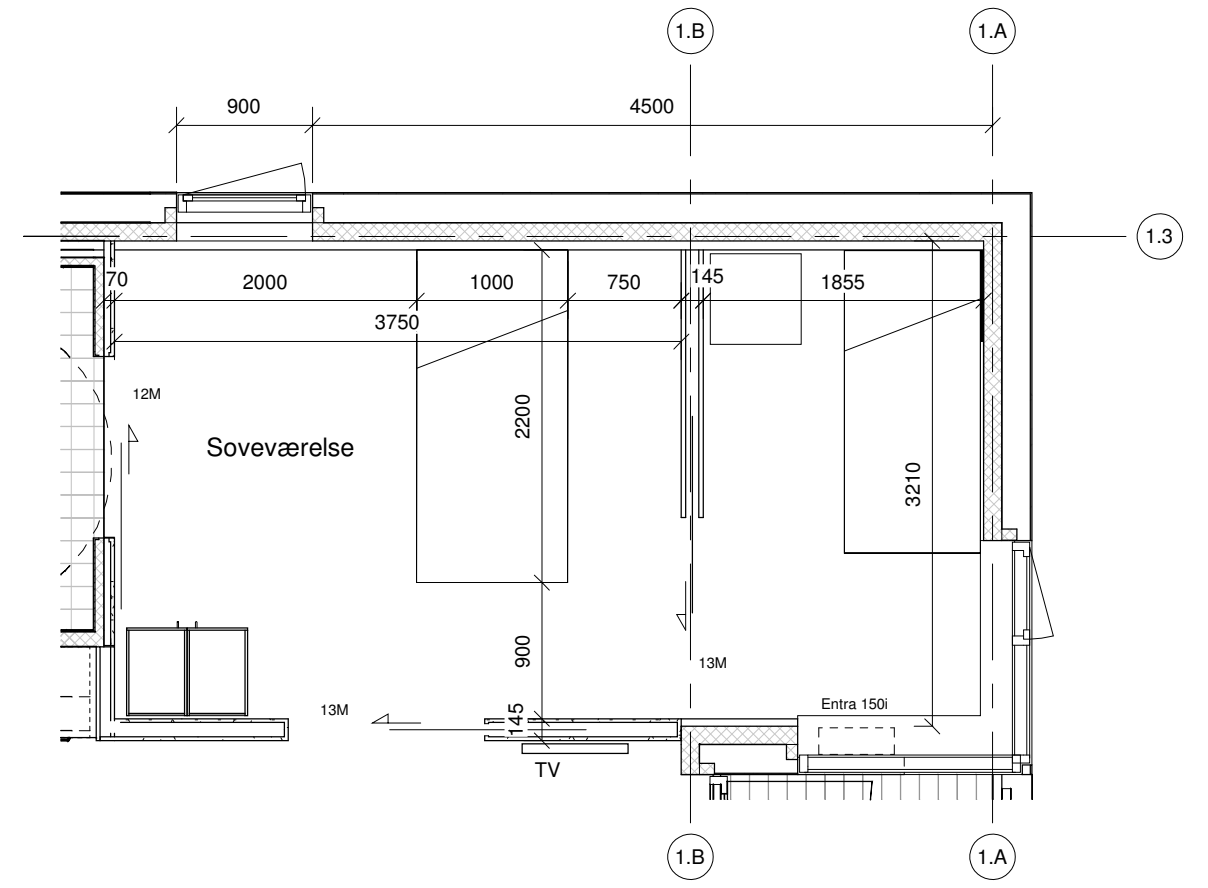
Bolig type 3 - ægteparbolig m. skillevæg
