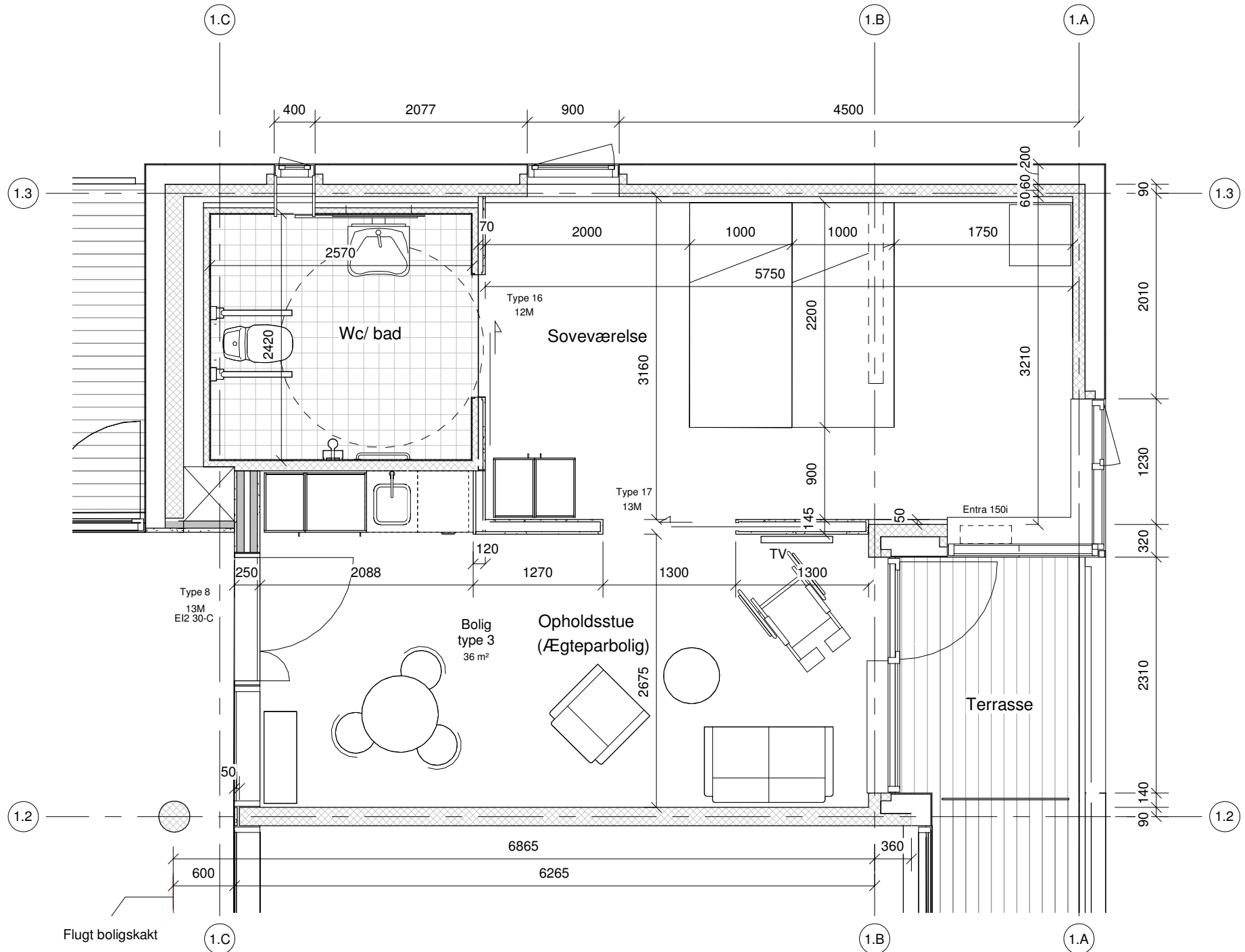
Bolig type 3 - ægteparbolig
