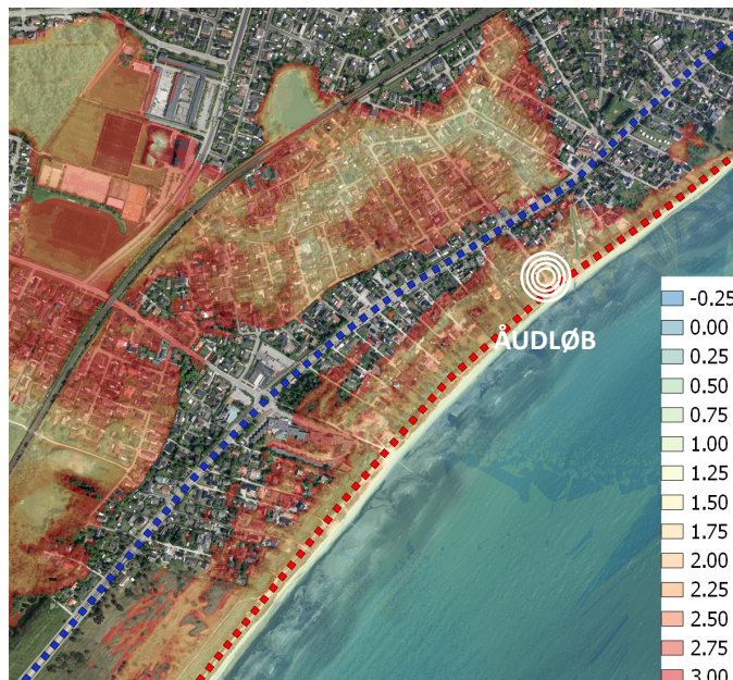
Differentieret sikring - blå linje er en sikring til kote 2,80 m mens rød linje er en sikring til kote 1,54 m. Højvandslukke i vandløb ved Oldermundsvej
