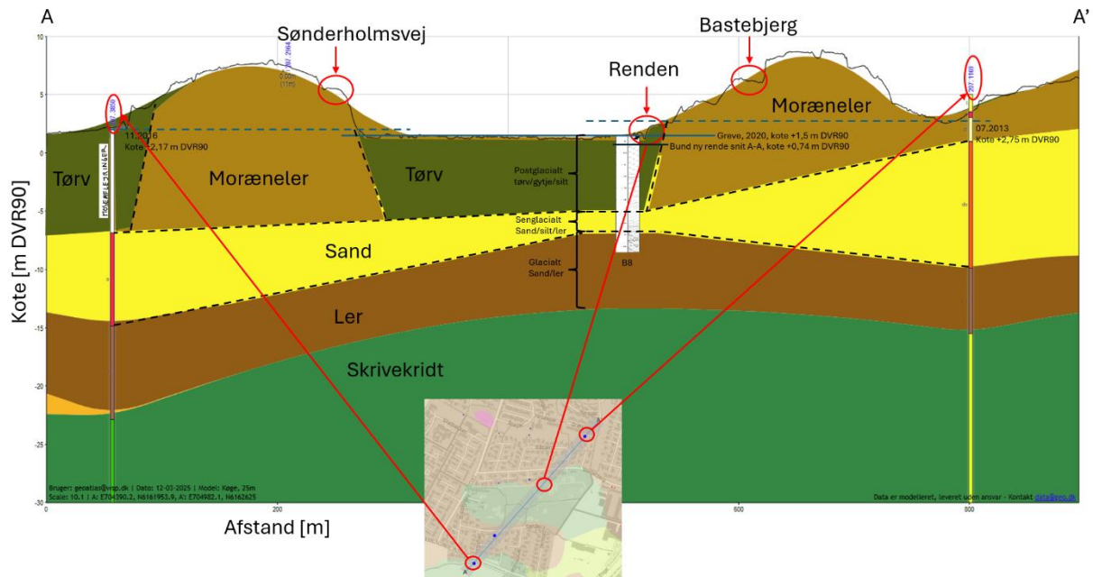
Figur 11-3. Konceptuelt geologisk tværsnit baseret på Geologisk model for Køge Bugt-området, 25 m (GEO Thomas Breum Andersen (TBA), 2019), tilrettet med den observeret geologi i borerne. Det ses, at kalken træffes nederst mellem kote -13 og -23 m DVR90. Over kalken er der et tilsyneladende gennemgående lag af ler, hvor oversiden træffes mellem kote -7 og -15 m DVR90. Over leret træffes et tilsyneladende gennemgående sandlag, hvor oversiden træffes mellem kote +1,5 og -7 m DVR90. Over sandlaget træffes der i Brødmosen postglaciale aflejringer i form af tørv mens forhøjningerne nord og syd for Brødmosen består af moræner. Der er blevet foretaget pejlinger af grundvandspotentialet i kalken samt udarbejdet et potentialekort for området (Figur 11-4)
