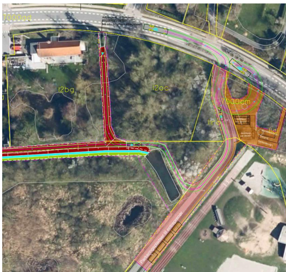
Figur 3-9 Adgangsvej til skurby/materialeplads fra Bastebjerg. Kørekurve med 12 m lastbil. Intern kørsel
