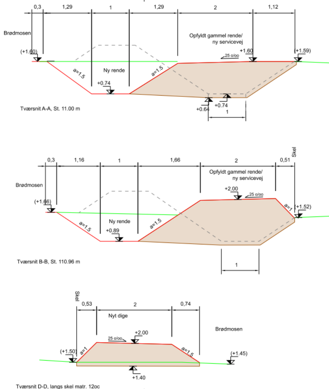
Figur 3-4 Eksempler på to tværsnit i st. 11.00 m (øverst), 110,96 m (miderst) og tværsnit D-D langs skel ved. Matr. 120c (nederst). Grøn streg er eksisterende terræn iht. den danske højdemodel. Brun markering er ny lerjord. Stiplet sort streg er projekt fra 1970. Alle koter er i m DVR90.
