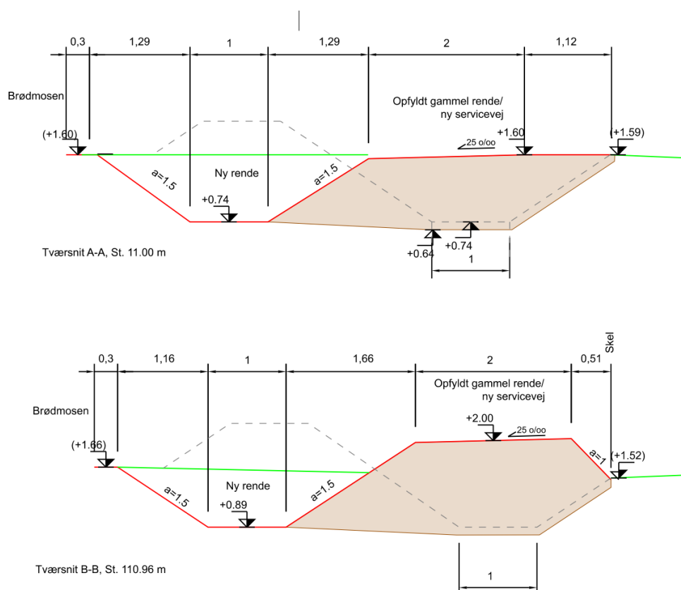
Figur 11-5. Tværsnit gennem fremtidigt dige. Det nuværende terrænforløb kan ses som stiplet grå linje. Det ses, at der byttes om på dige og rende og at rendens bundkote fastholdes. Kilde: (WSP, 2024)
