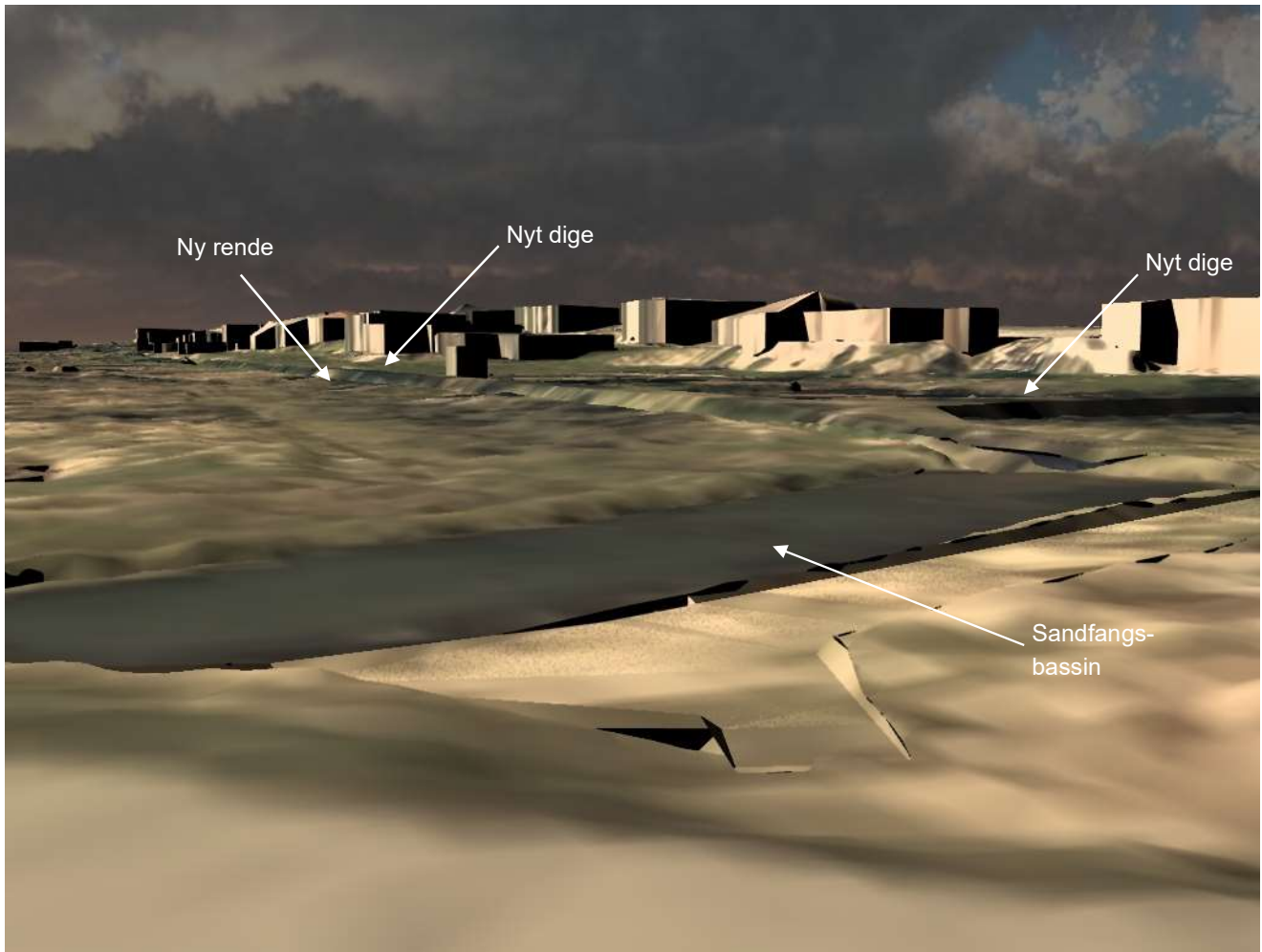
Visualisering 3. Nyt dige og forlagt rende set fra øst mod vest. Sandfangsbassin i forgrunden.
