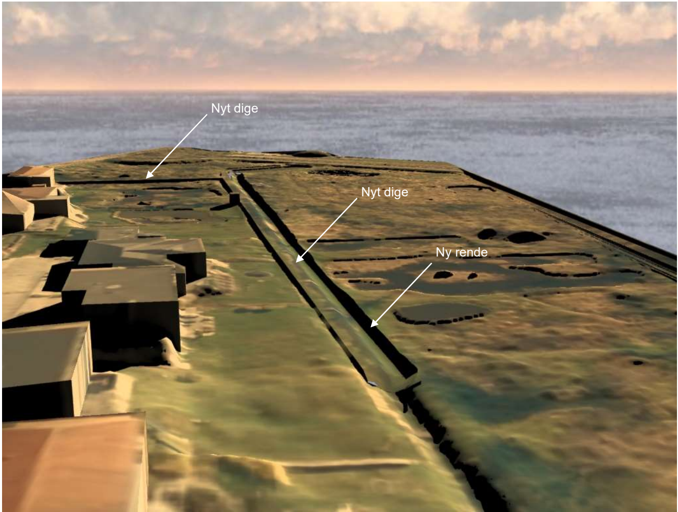
Visualisering 4. Nyt dige og forlagt rende set fra vest mod øst.
