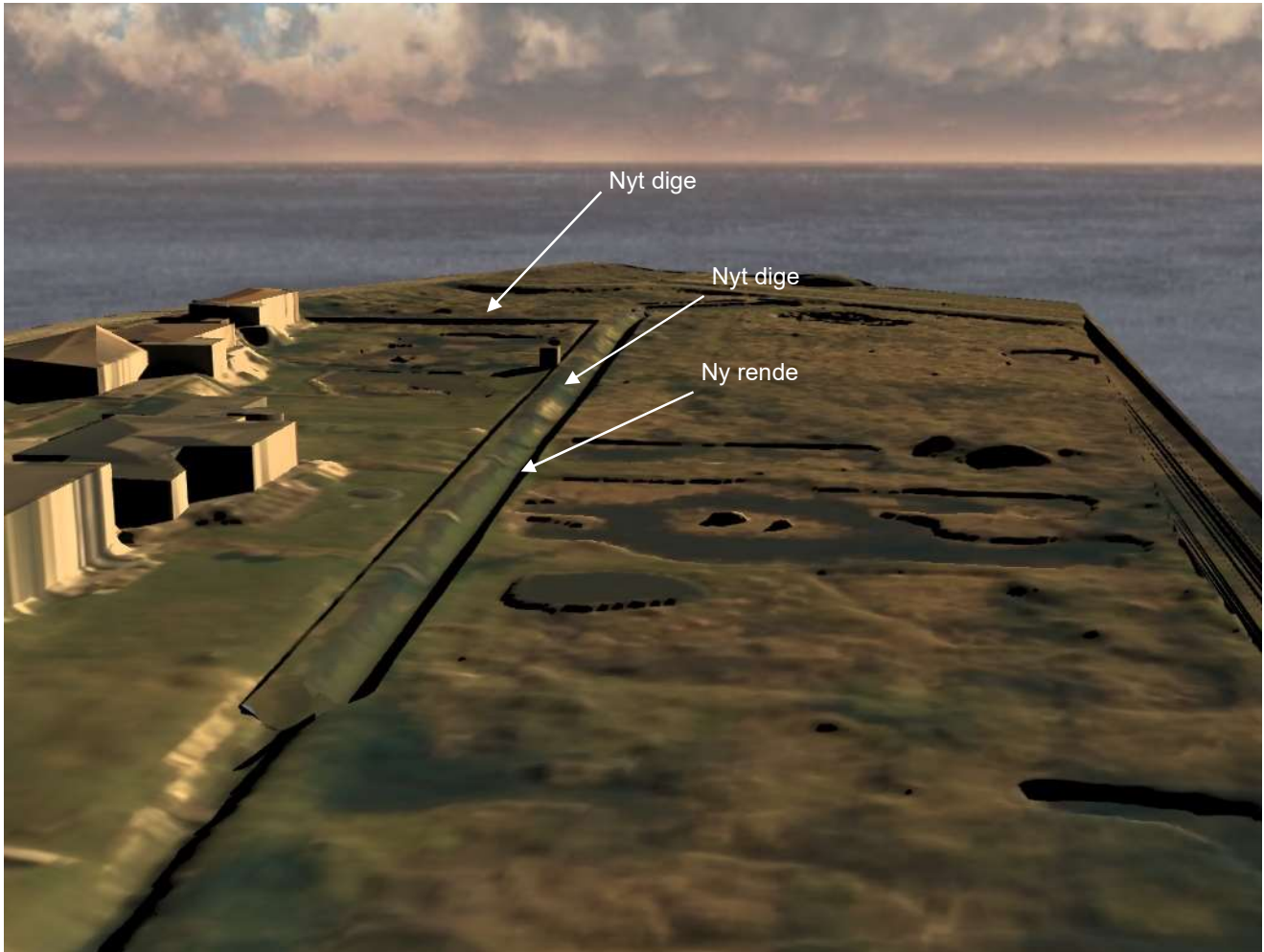
Visualisering 5. Nyt dige og forlagt rende set fra vest mod øst.
