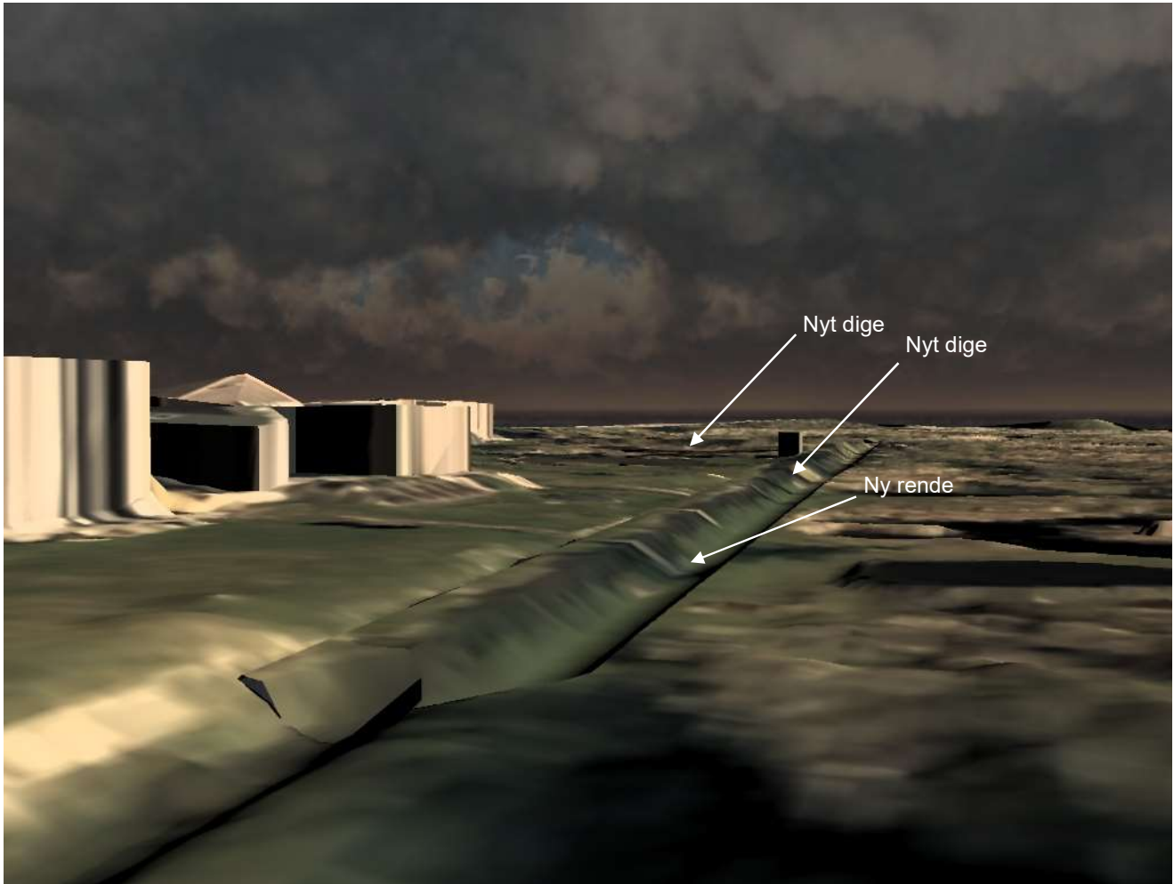
Visualisering 2. Nyt dige og forlagt rende set fra vest mod øst.
