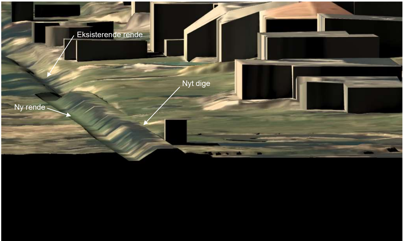
Visualisering 7. Nyt dige og forlagt rende set fra øst mod vest.
