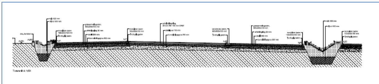
Figur 2: Eksempel på opbygning af p-plader på græsarmeringssten med afvanding til forsinkelsesvolumen i regnbede/grøfter med filtermuld.
